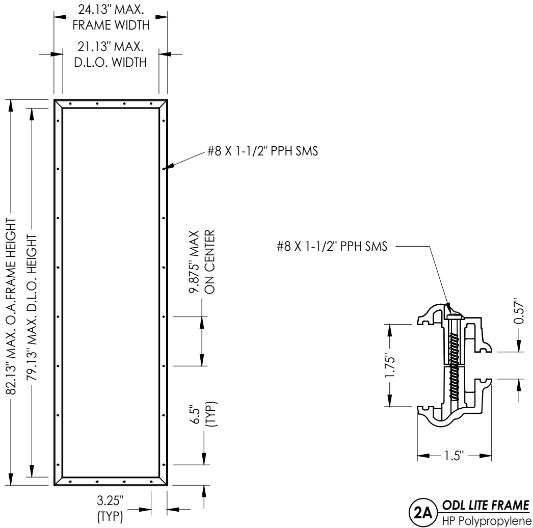
ODL LITE FRAME
